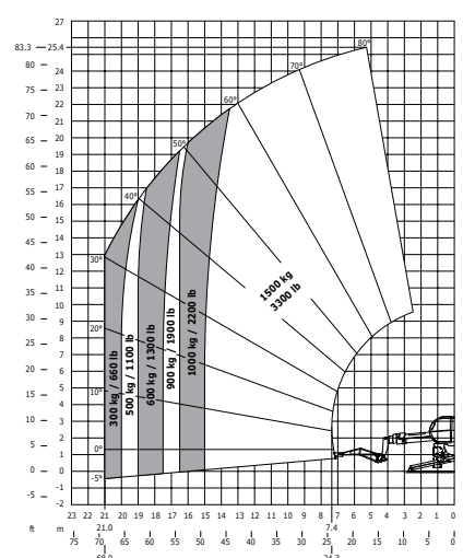
Rotazione su stabilizzatori estesi con braccetto 1500 kg EN 1459
